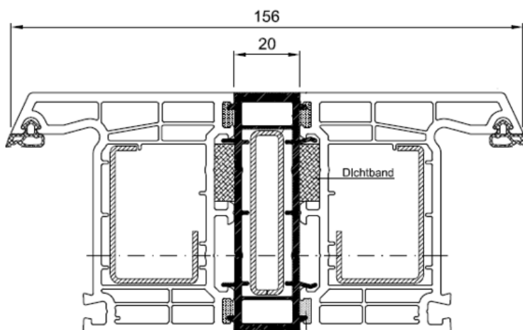
Obr. 42b. Príklad spojenia okien z PVC profilov
