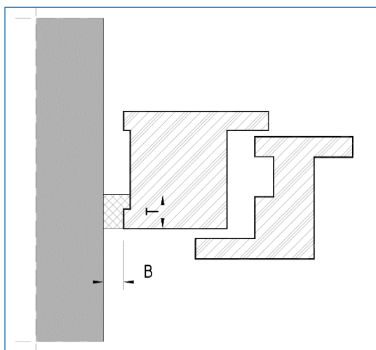
Obr. 15. Rozmery tesnenia z impregnovaných parotesných expanzných pásov
